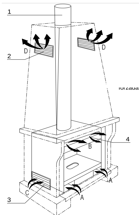
1-Tuyau cheminée 2-Bouches d'air chaud 3-Bouches d'air froid 4-Sortie convection forcée
